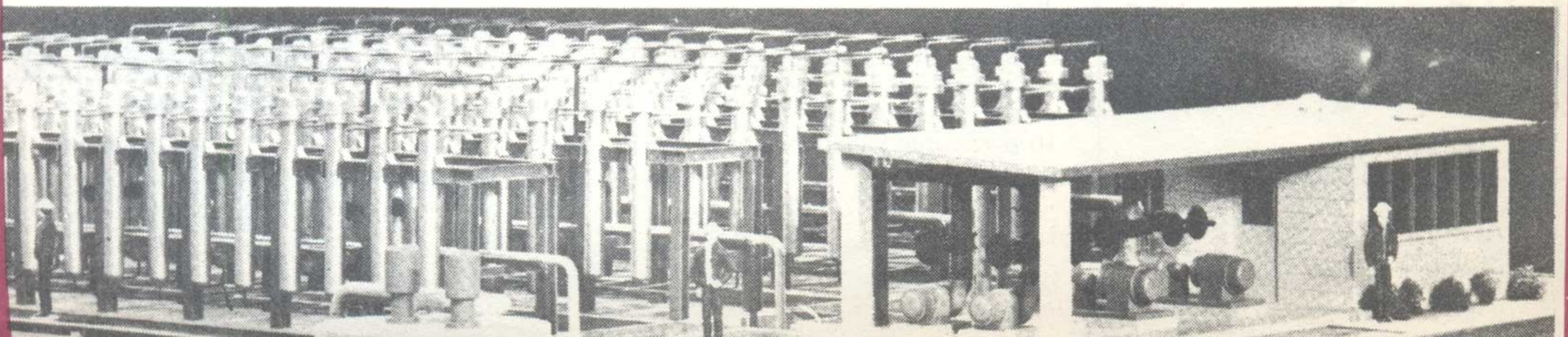
Planta modelo de purificación de agua por el proceso ósmosis inversa, proyectada por Dupont.
